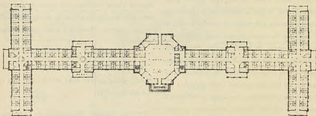
Fig. 2. — Hospital Henry Ford a Detroit, Michigan. Plànol de la planta baixa.
