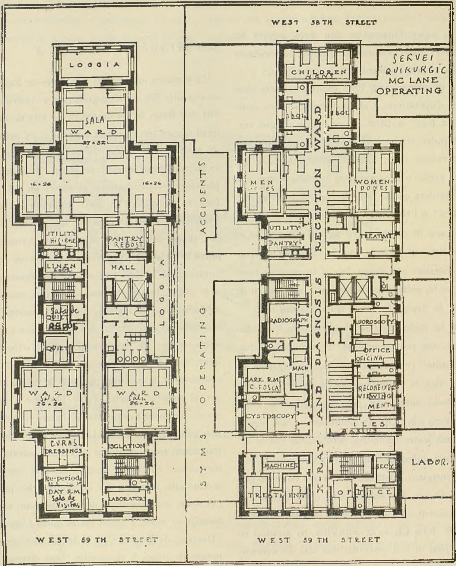
Fig. 4. — Hospital Roosevelt a New York City. Nou pabelló. A.—Plànol d'un dels pisos superiors. B.—Plànol de la planta baixa.
