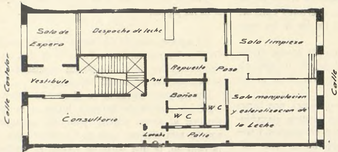
Planta baixa
