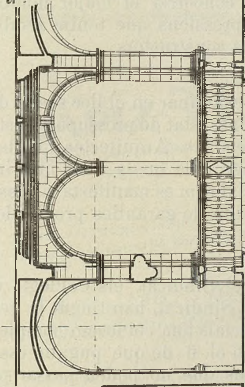
Casal del Metge - Detalls de la entrada i hall central -
