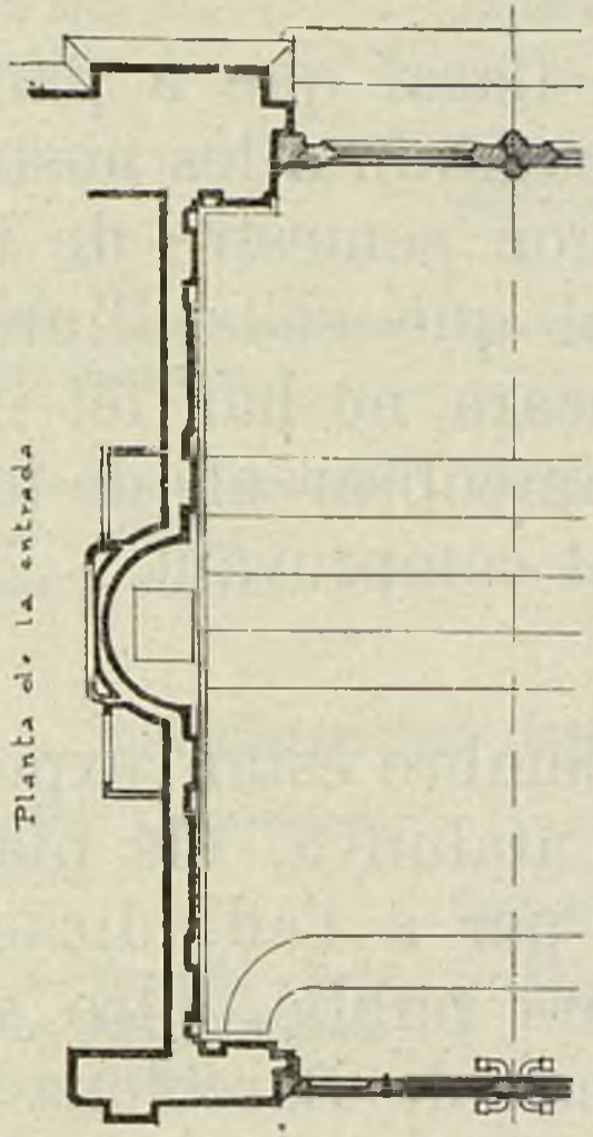
Casal del Metge - Detalls de la entrada i hall central -
